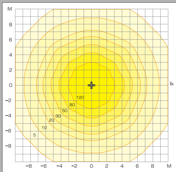
Диаграмма освещенности для QU38 Площадка 20 x 20 метров
