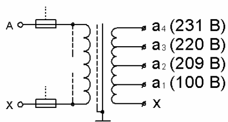
Принципиальная схема трансформатора
