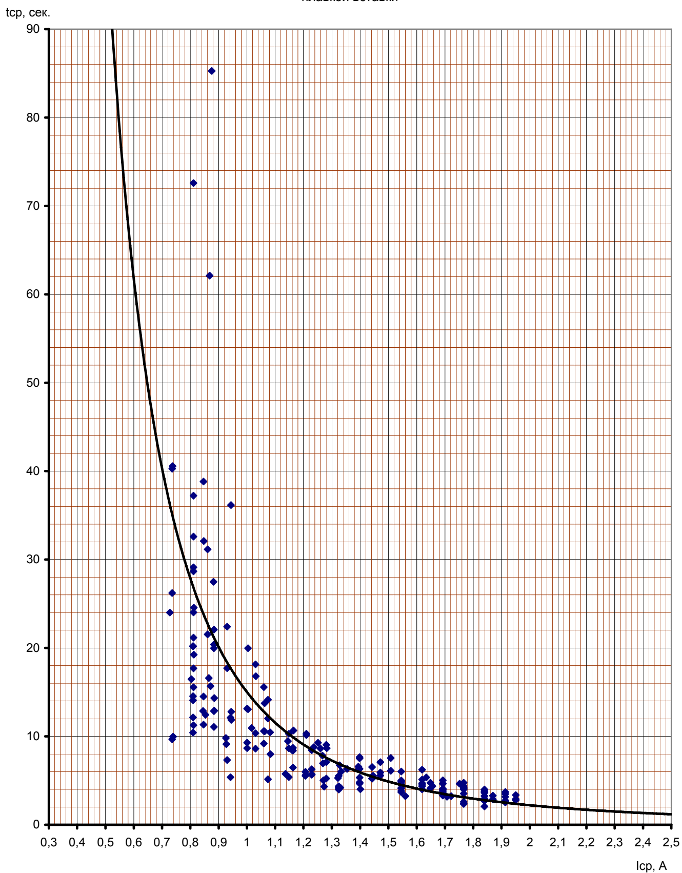
Продолжение приложения А Рисунок А.3 Ампер-секундная характеристика защитного предохранительного устройства с резистором С2-33-Н-0,25 6 Ом для трансформатора ОЛСП-1,25/6 в качестве плавкой вставки
