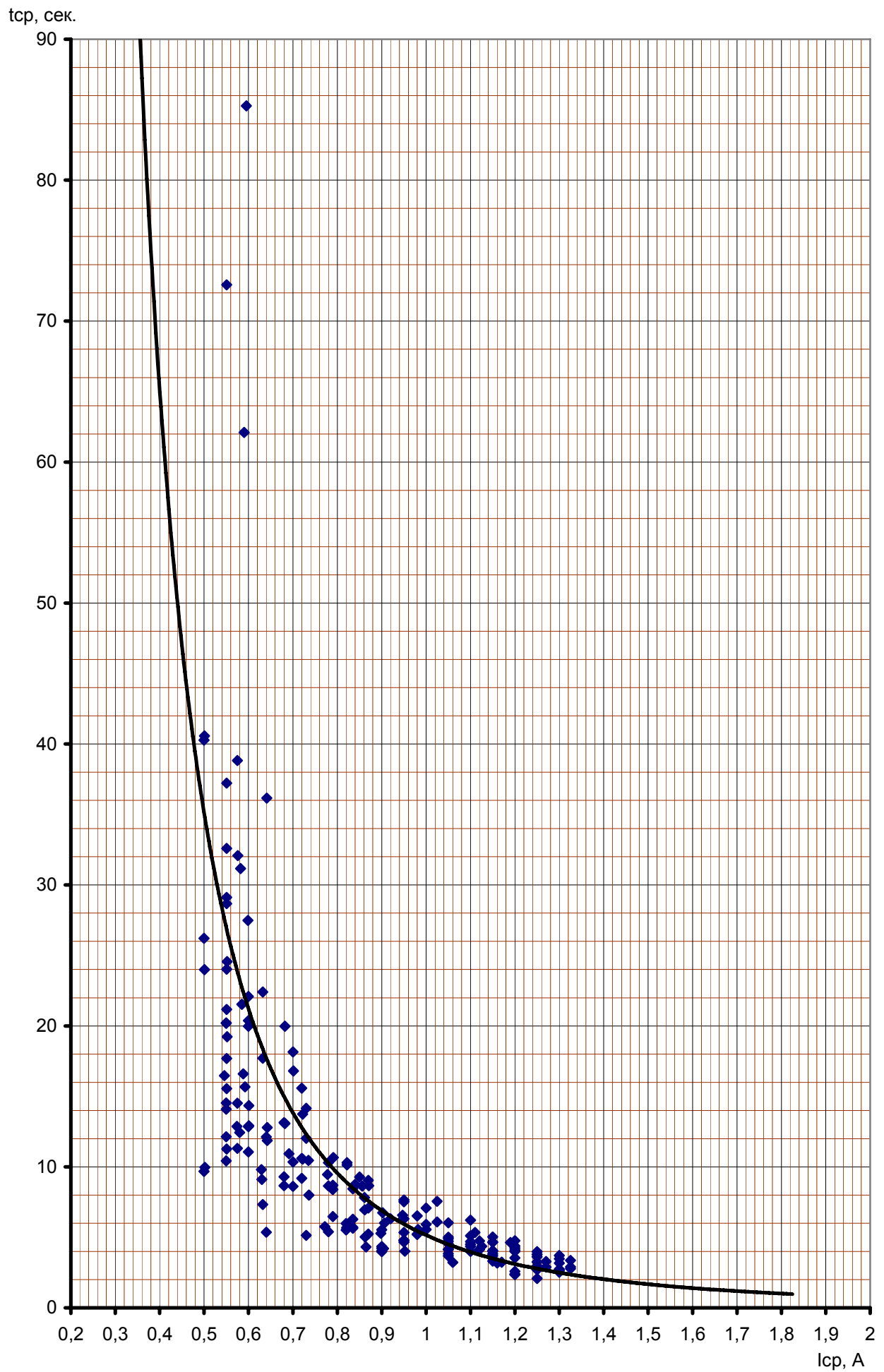
Рисунок А.4 Ампер-секундная характеристика защитного предохранительного устройства с резистором С2-33-Н-0,25 13 Ом для трансформатора ОЛСП-1,25/10 в качестве плавкой вставки.
