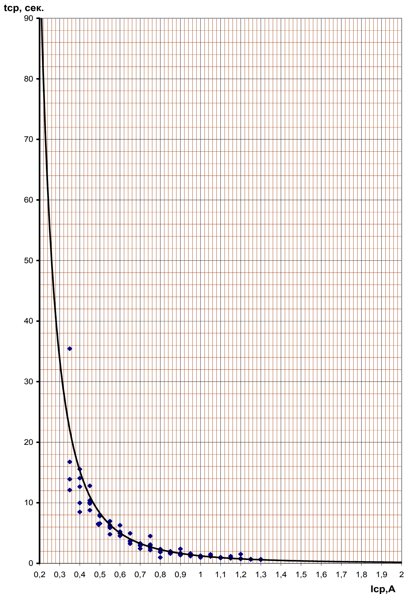
Рисунок А.2 Ампер-секундная характеристика защитного предохранительного устройства с резистором С2-33-Н-0,25 36 Ом или С2-33-Н-0,125 18 Ом для трансформатора ОЛСП-0,63/10 в качестве плавкой вставки.
