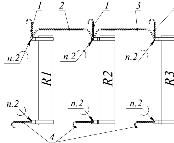
Рисунок Б.2 Монтажная схема соединения резисторов
