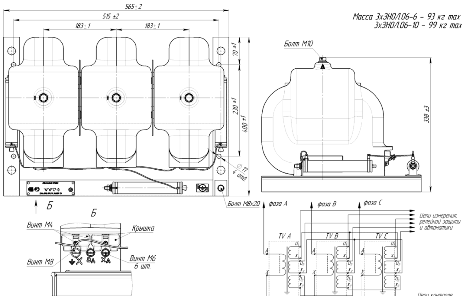
Рисунок А.3 Общий вид трехфазной группы 3хЗНОЛ.06
