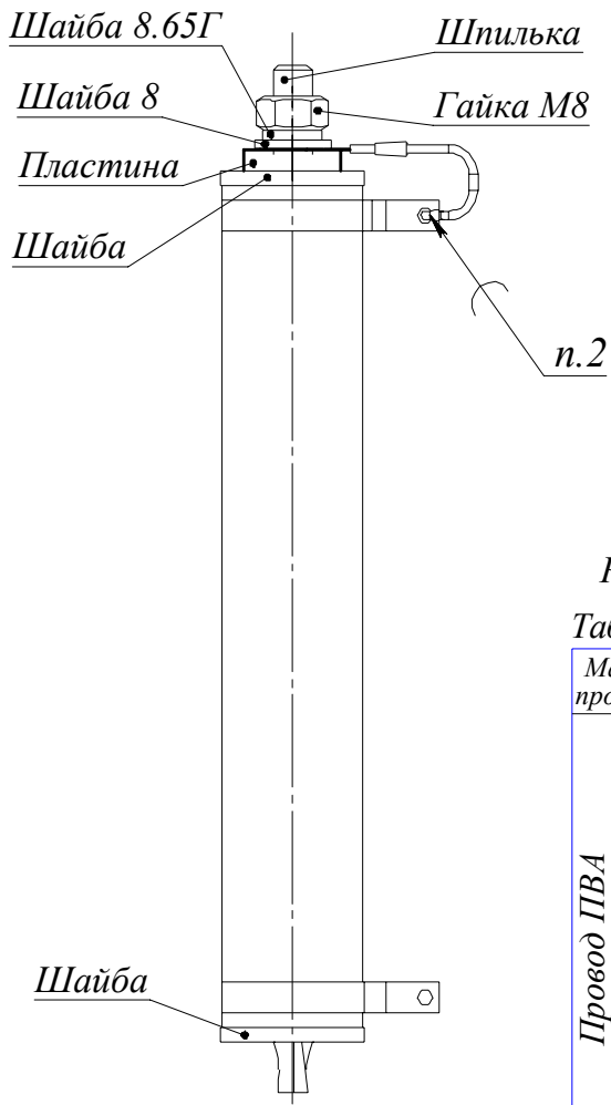
Рисунок Б.1 Установка резистора
