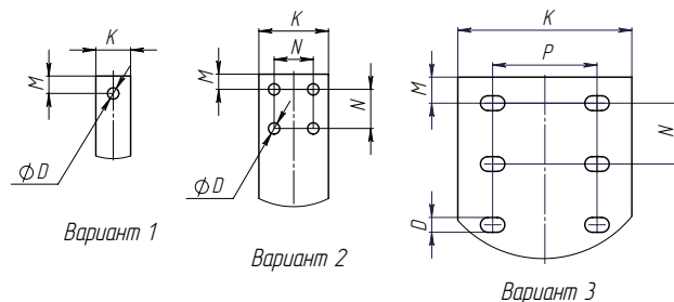
Рис. 5. Варианты исполнения шин НН для трансформаторов ТЛС-100...3150
