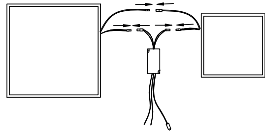
1. Схема подключения элементов плафона
