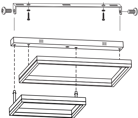
2. Схема крепления плафона к основанию
