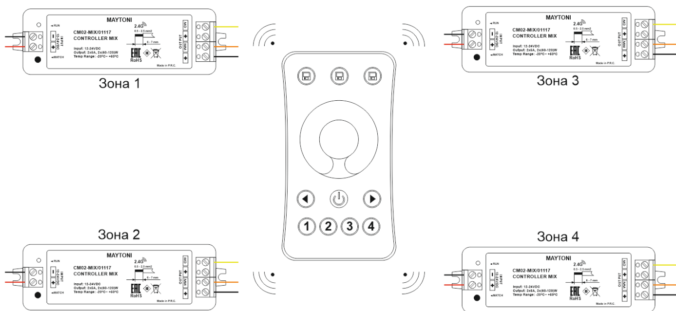
Рис. 3 разветвленная система с многозонным пультом управления
