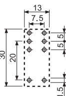
95.15.2 Вид сбоку
