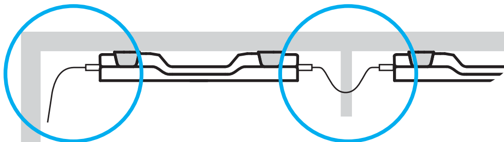
Подключение до 7 светильников последовательно
