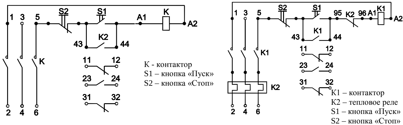
Пускатели нереверсивные без реле, с встроенными в оболочку кнопками управления, с 2з+2р контактами вспомогательной цепи
