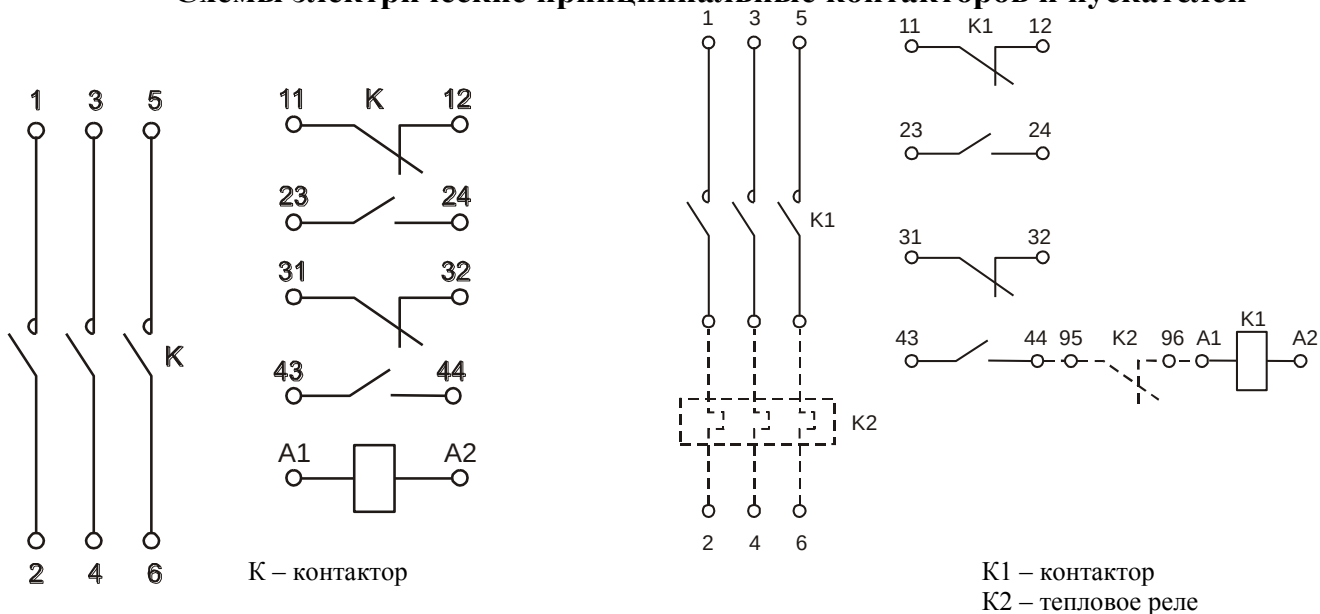
Контакты нереверсивные с 2з+2р контактами вспомогательной цепи
