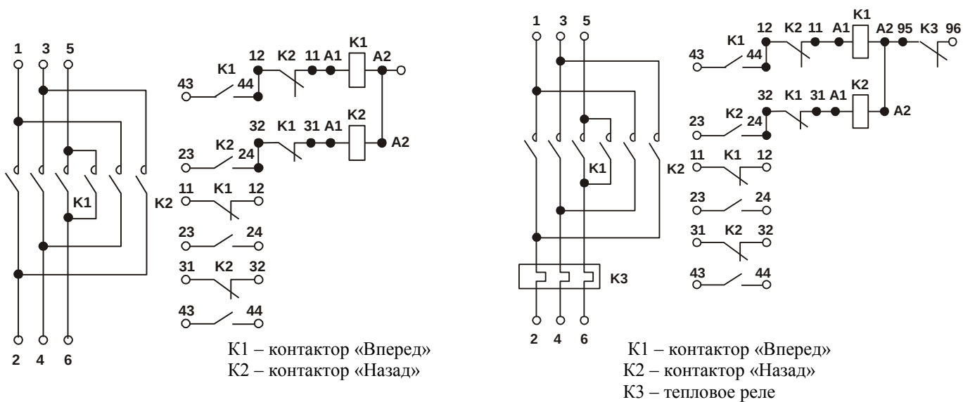
Контакты реверсивные без реле, с 4з+4р контактами вспомогательной цепи
