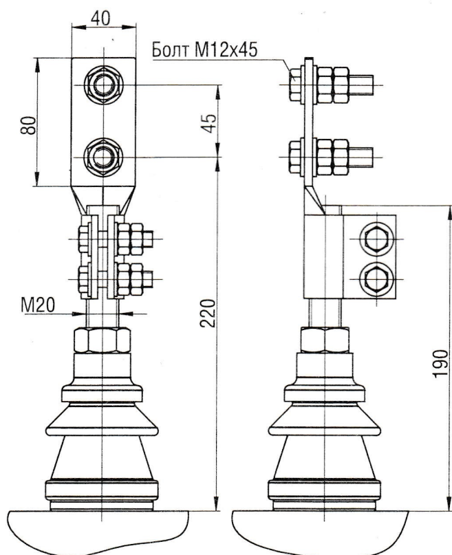
ввод НН на номинальный ток 630 А
