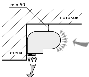
Схема настенного монтажа завесы «Мини-3»
