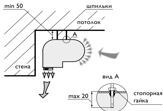
Схема расположения мест крепления завес «Мини-3»
