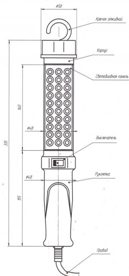
Переносной светодиодный светильник типа СРП.
