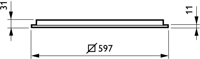
Чертеж размеров
