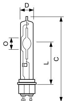
CDM TMW 210W/930 PGZ18 U
