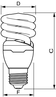
QSPIR-F 15W/827 E27 220-240V 50/60Hz
