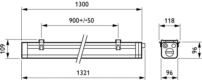
Чертеж размеров
