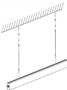
Рис.2. Монтажный чертёж.
