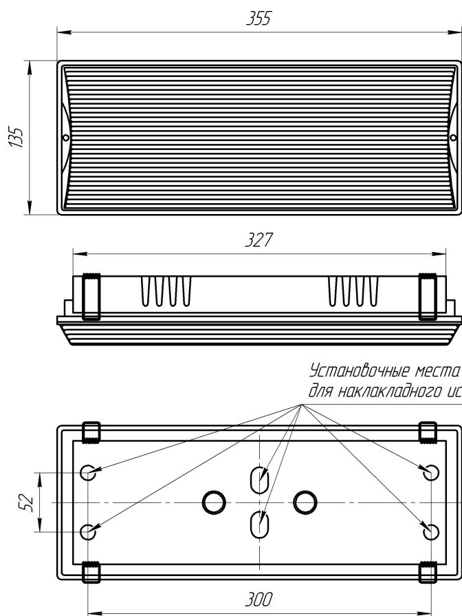
Рис. 1. Габаритные размеры
