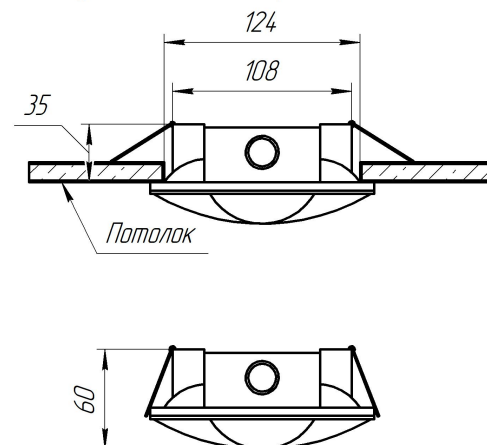
Схема установки для встраиваемого исполнения
