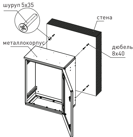
Рис. 1.1. Схема настенного монтажа.
