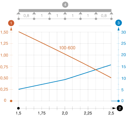
Диаграмма нагрузки
