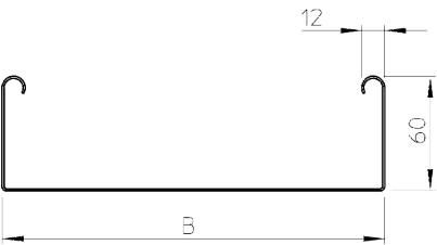
Размеры
