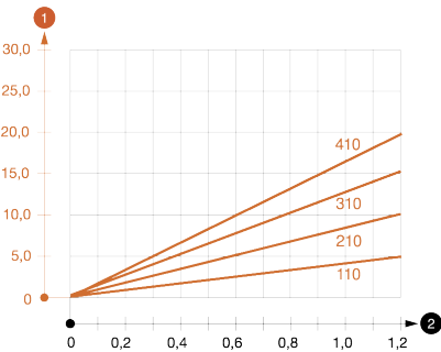
Диаграмма нагрузки
