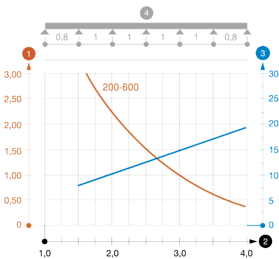
Диаграмма нагрузки
