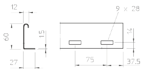
Размеры
