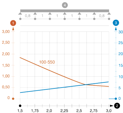
Диаграмма нагрузки
