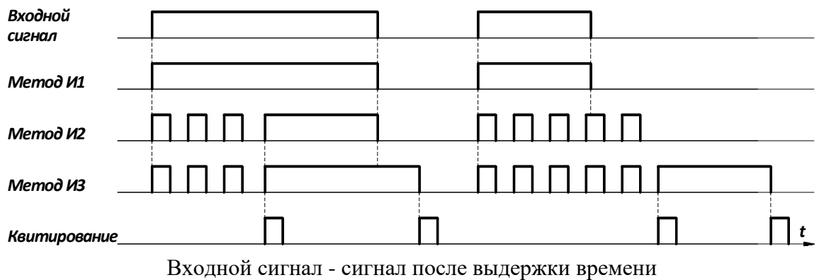
Рисунок 4 - Временные диаграммы управления индикацией
