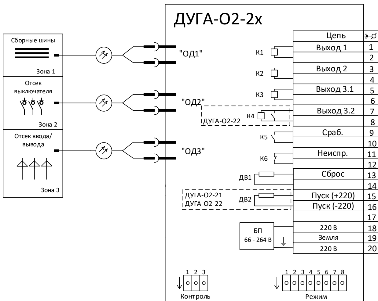
Рисунок 3 - Схема электрическая подключения с ЦОВ
