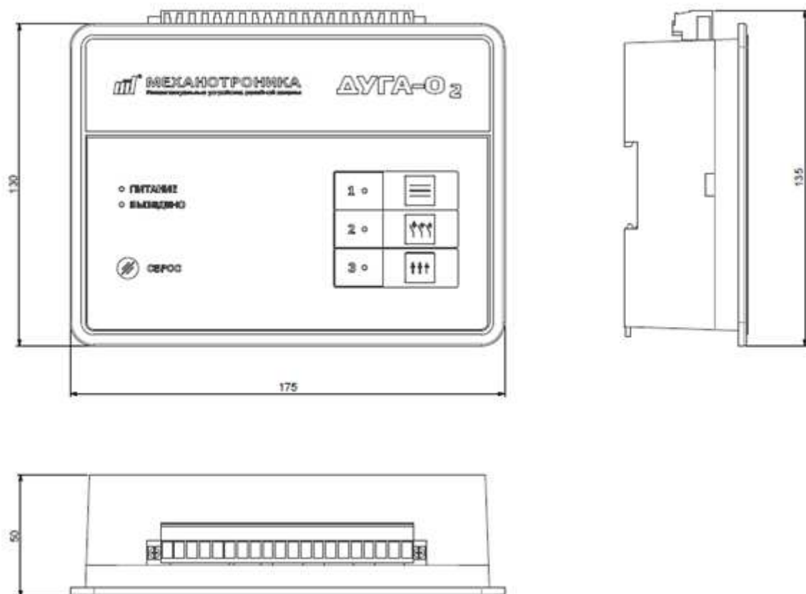
Рисунок 1 – Габаритные и присоединительные размеры регистратора
