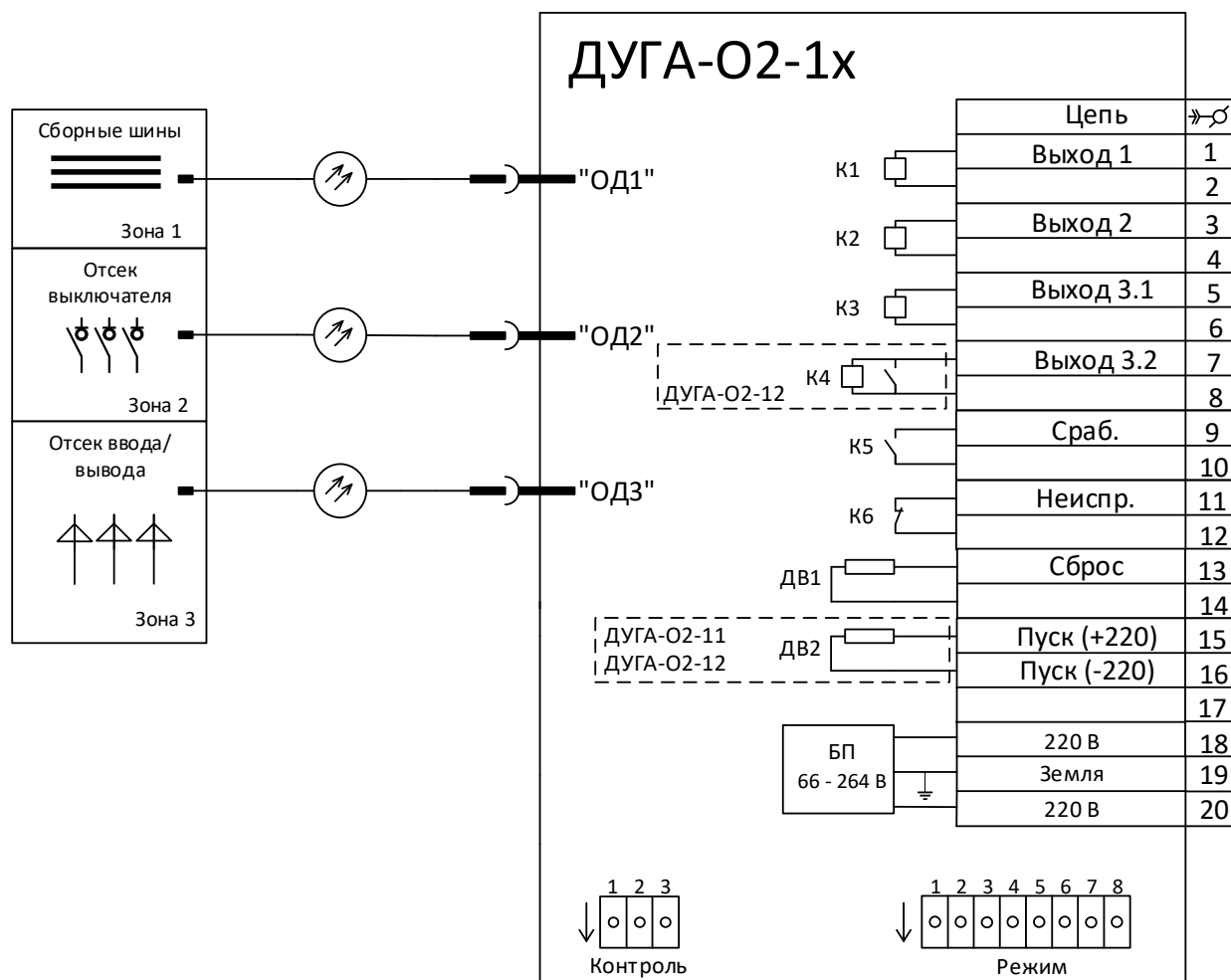
Рисунок 4 - Схема электрическая подключения без ЦОВ
