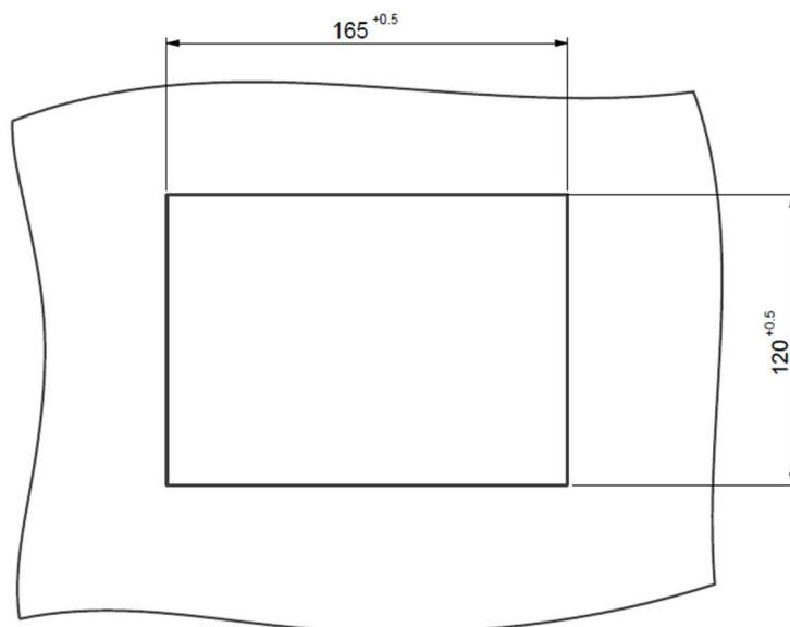
Рисунок 2 - Разметка для крепления регистратора
