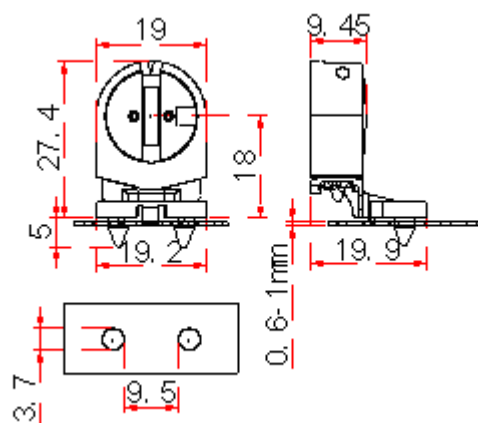
Патрон (ламподержатель) G5, вставной с лицевой стороны, h-оси 18mm, для люминесцентной лампы T5, (крепление на цапфы)
