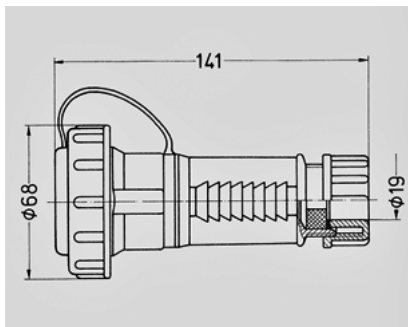
Чертеж 3 МВ 41 Размеры, мм.
