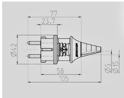
Чертеж 2 МВ 139 Размеры, мм.
