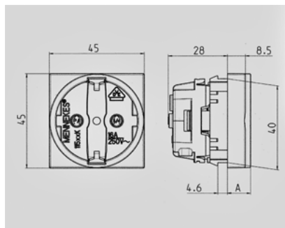
Чертеж 1 MB 457 Размеры, мм.
