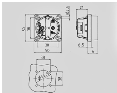
Чертеж 1 МВ 450 Размеры, мм.
