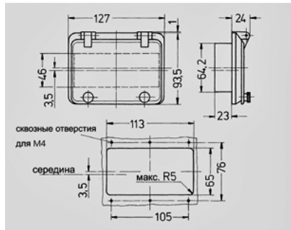
Чертеж 6 МВ 17
