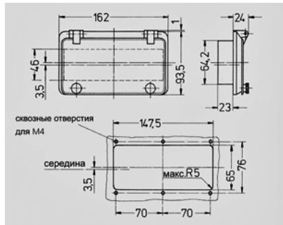
Чертеж 6 МВ 12
