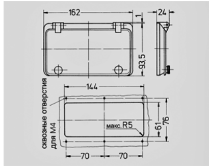
Чертеж 6 МВ 15
