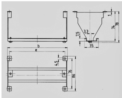
Чертеж 6 МВ 18
