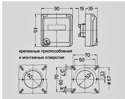
Чертеж 1 MB 305
