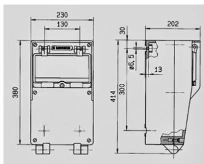
Чертеж 5 МВ 42 Размеры, мм.
