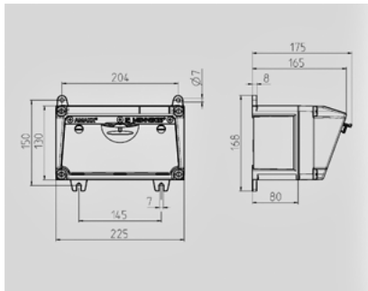
Чертеж 1 MB 531
