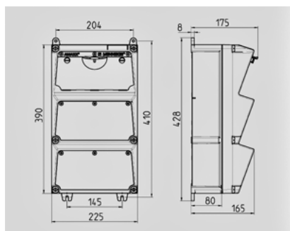
Чертеж 1 MB 522
