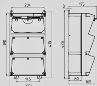
Чертеж 1 MB 522
