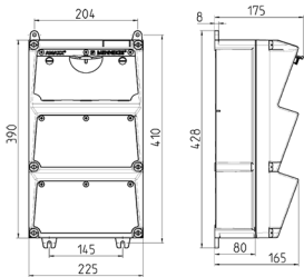
Чертеж 1 MB 522
