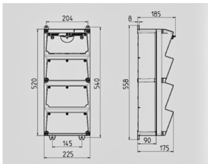
Чертеж 1 MB 523
