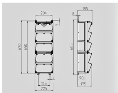
Чертеж 1 MB 540
