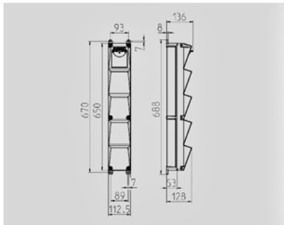
Чертеж 1 MB 541
