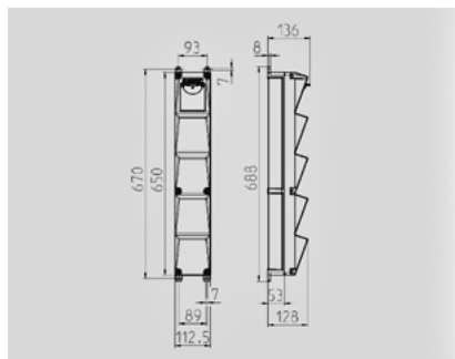
Чертеж 1 MB 541
