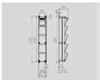
Чертеж 1 MB 541
