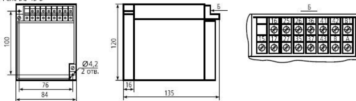
Реле ВС-43-3
