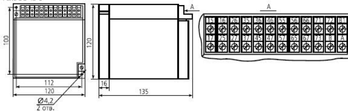
Реле ВС-43-6
